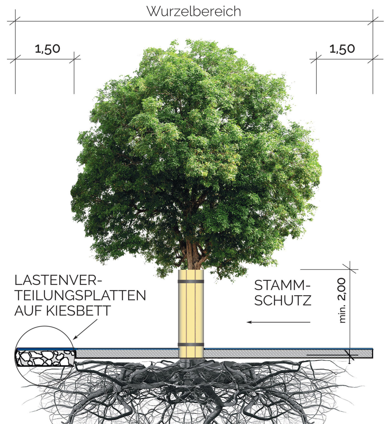
WURZELSCHUTZ DURCH LASTENVERTEILUNG
